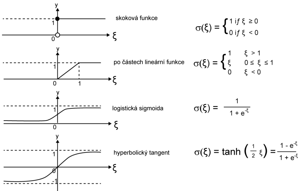
Obr. 7 Aktivační přenosové funkce.
