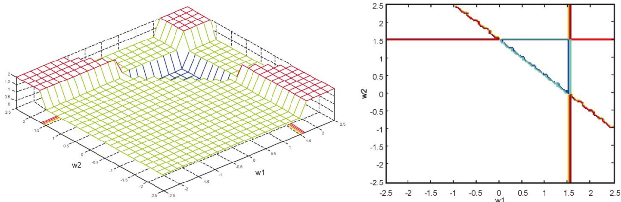
Obr. 11 Grafické řešení nastavení vah neuronu pro realizaci funkce AND.
